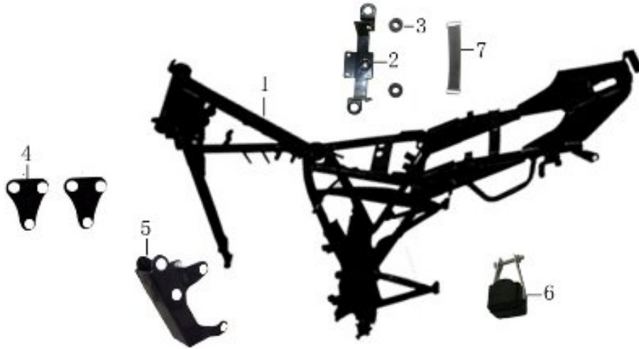
F-20 车架焊接总成 MAIN FRAME WELDMENT
